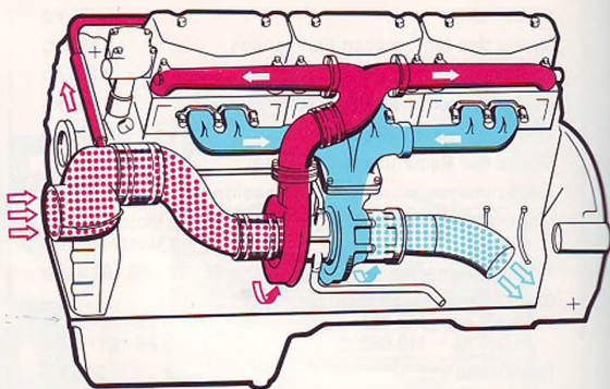
Turbolader • Saugseite • Auspuff
