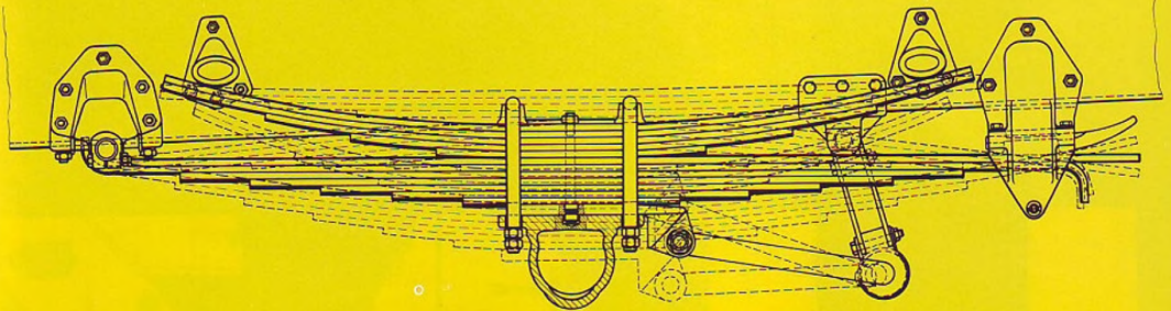
Federung der Hinterachse
