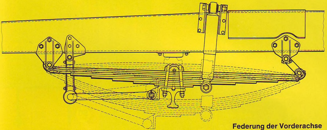
Federung der Vorderachse
