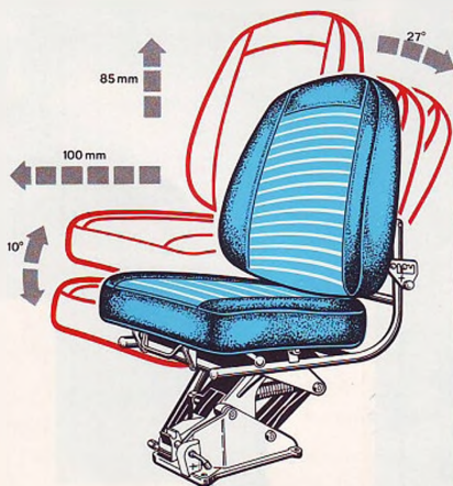
Einstellmöglichkeiten und Federung
