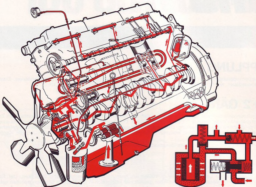
Schema der Motorschmierung
