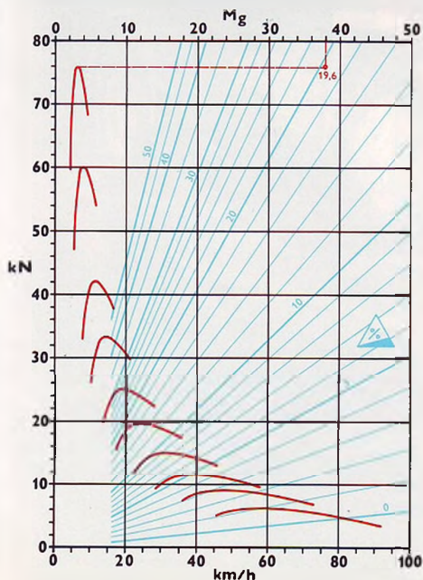
Steigfähigkeit des vollbelasteten Zuges
