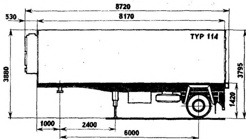
Схема полуприцепа-рефрижератора Н13Х типа 114
