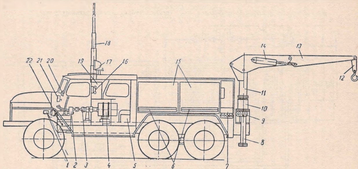
Рис. 2. Компонка основных агрегатов автомобиля технической службы, связи и освещения:
