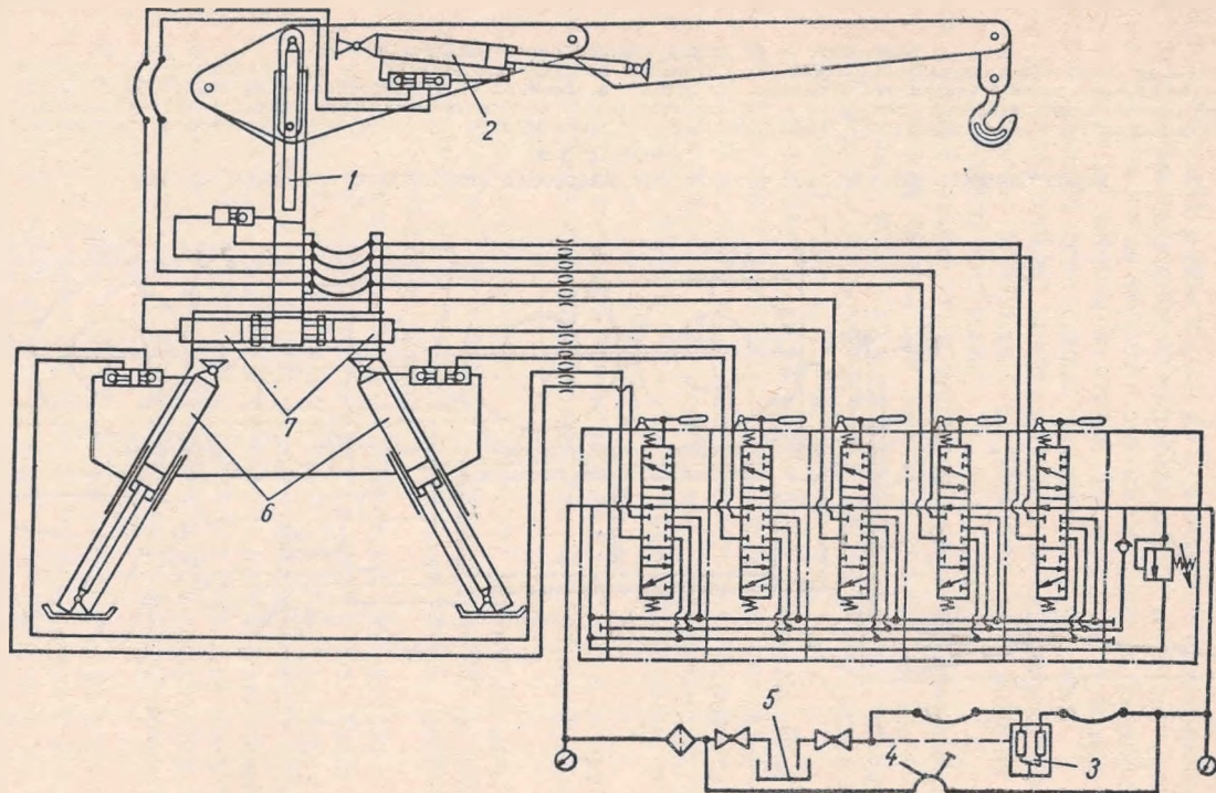
Рис. 3. Принципиальная гидравлическая схема автомобиля технической службы, связи и освещения АТСО-20(375):
