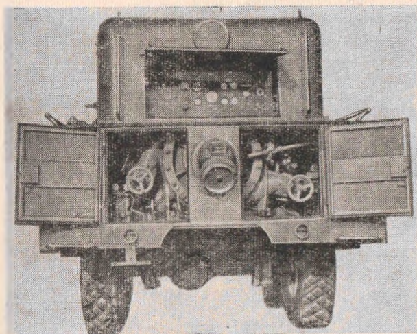
Рис. 1. Станция пожарная насосная ПНС-110(131), модель 131:
