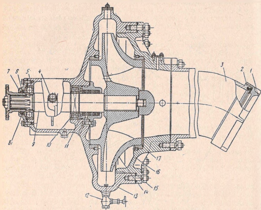
Рис. 3. Насос пожарный ПН-110:
