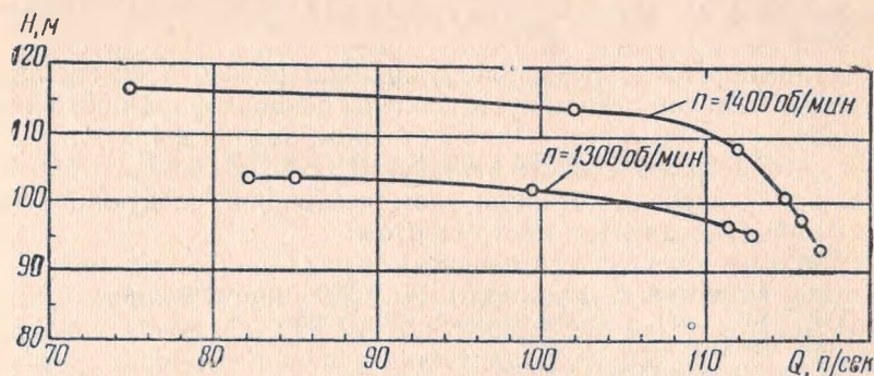
Рис. 4. Рабочая характеристика насоса ПН-110
