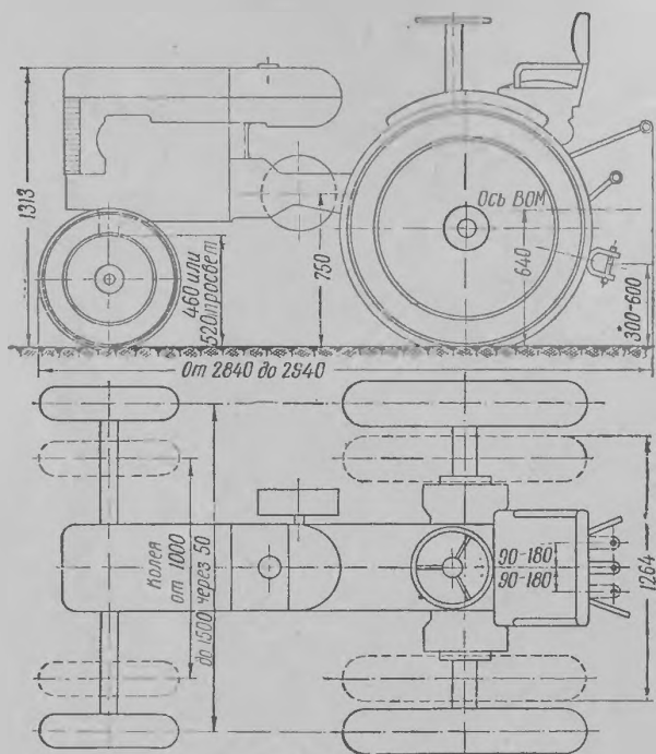
Рис. 14. Схема трактора ХТЗ-7, наладенного для выполнения междурядных работ (наладки А и Г).
