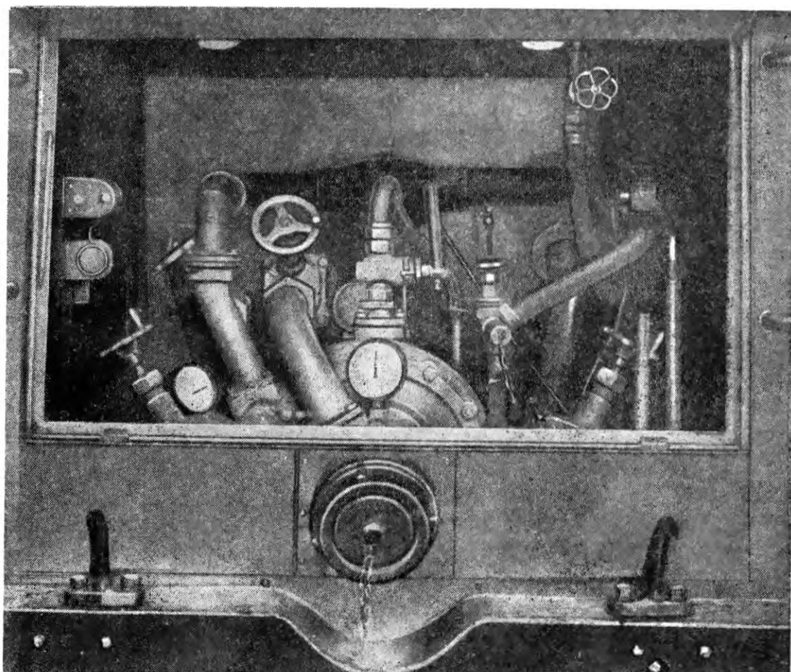
■ Рис. 28. Насосный отсек автоцистерны АЦ-30(205)
