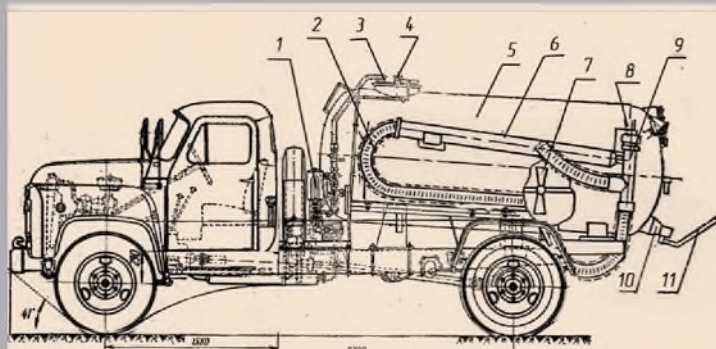
Общий вид автомобильного жидкеразбрасывателя РЖУ-3,6:
