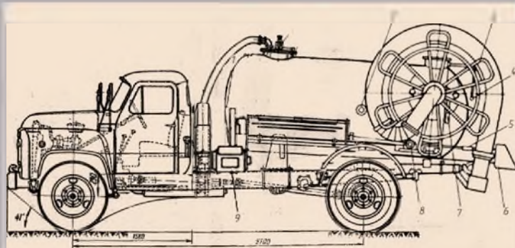
Общий вид вакуум-машины УК-19:
