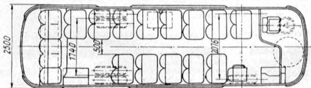
Схема автобуса ЛАЗ-695Б «Львов»
