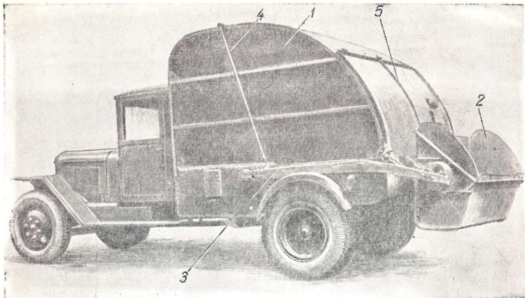
Рис. 340. Мусоровоз МС-1 на шасси автомобиля ЗИС-5:
