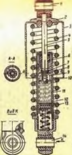
Рис. 143. Амортизатор задней подвески мотороллера Т-200:
