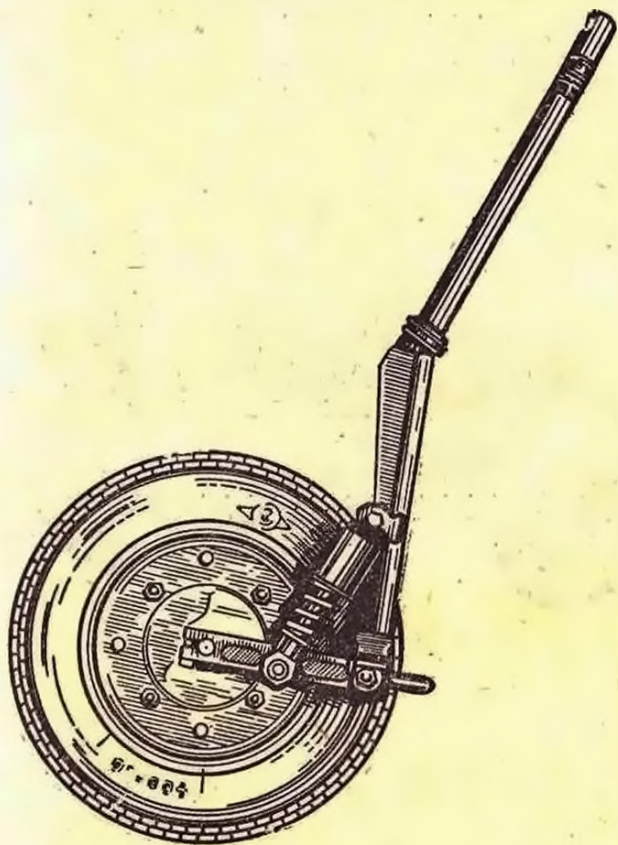
Рис. 147. Передняя вилка мотороллера Т-200М.
