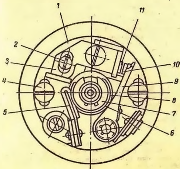
Рис. 137. Прерыватель мотороллера „Тула“:
