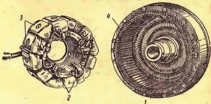
Рис. 136. Династартер мотороллера „Тула“:
