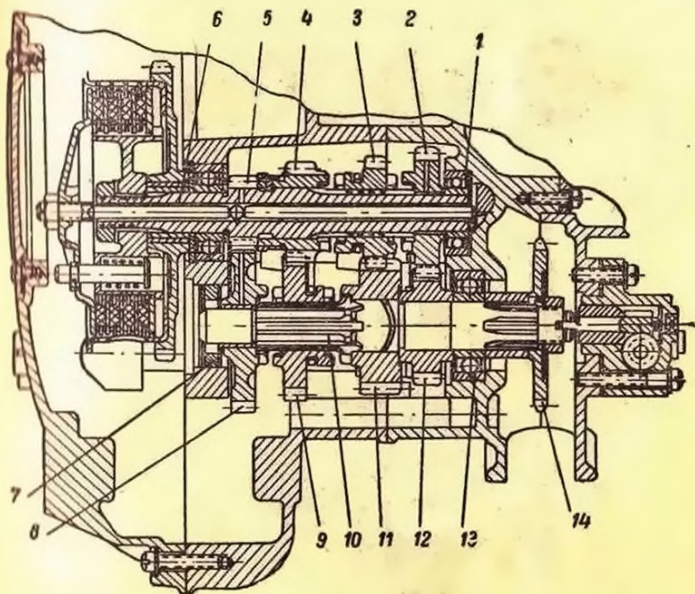
Рис. 141. Коробка передач мотороллера Т-200:
