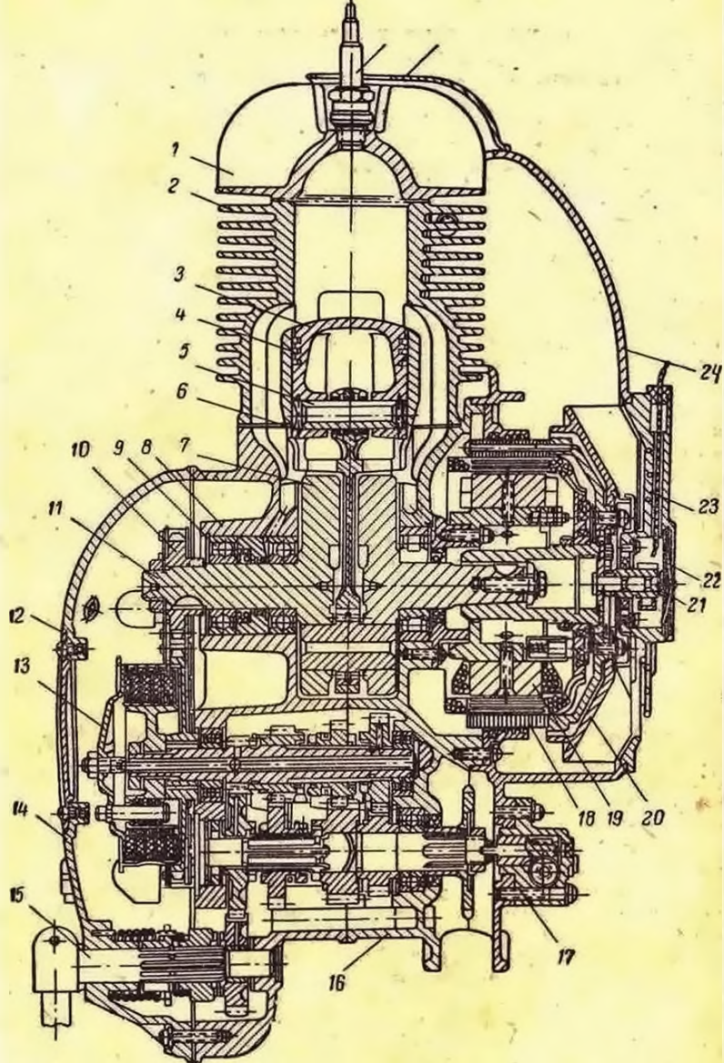
Рис. 133. Двигатель мотороллера „Тула“:
