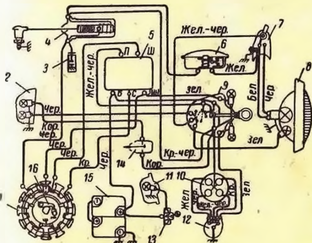
Рис. 139. Схема электрооборудования мотороллера Т-200:
