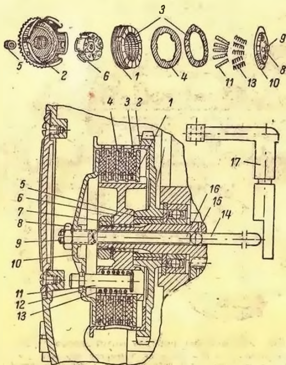
Рис. 140. Сцепление мотороллера Т-200:
