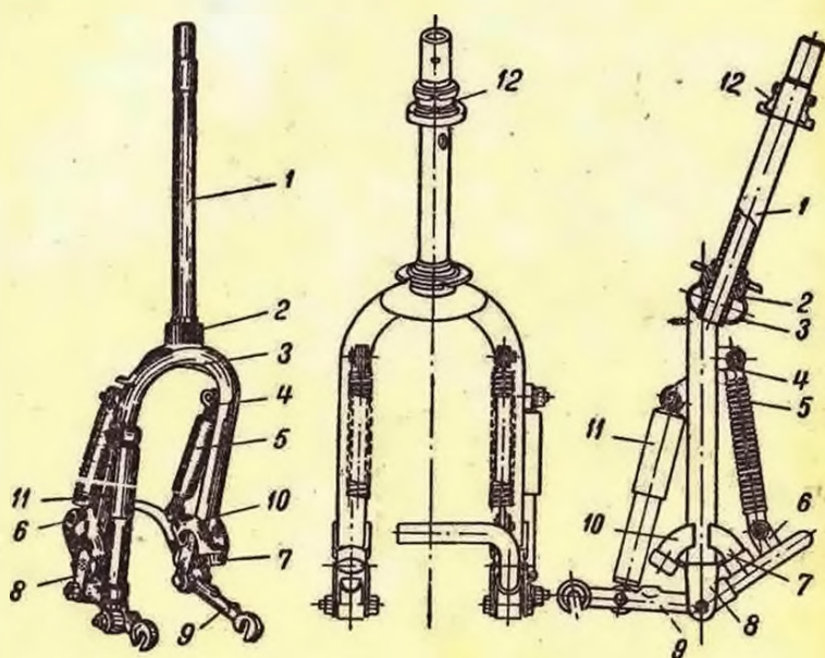
Рис. 142. Передняя вилка мотороллера „Тула“:
