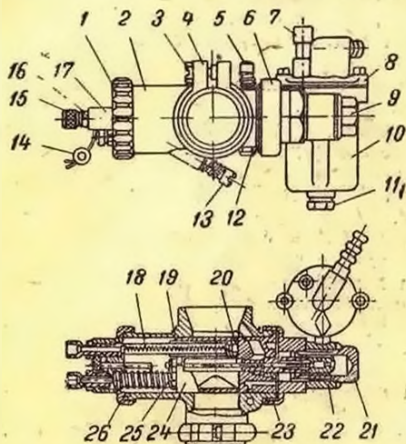
Рис. 134. Карбюратор К-28Г:
