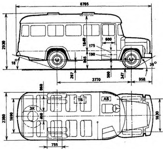
Автобус КАВЗ-3976 4×2.2
