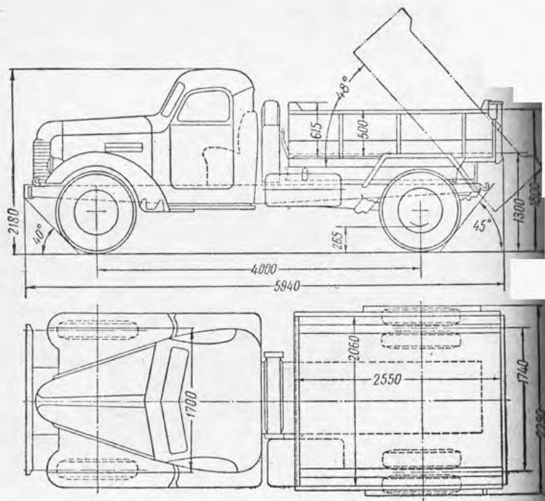
Рис. 101. Схема автомобиля-самосвала ЗИЛ-ММЗ-585М.
