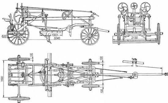
Рис. 1.7. Грейдер «Беджер» (1930)
