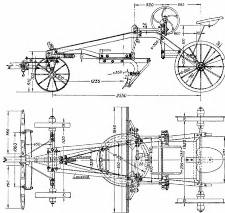
Рис. 1.6. Грейдер «Патруль» (1929)
