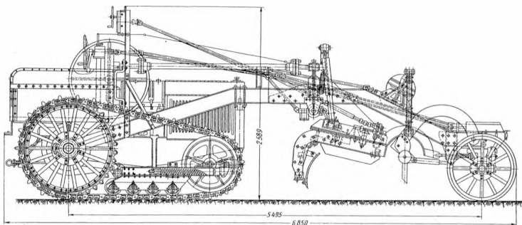
Рис. 1.10. Автогрейдер ЦДОРМАШНИИ (1934)
