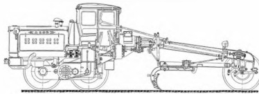
Рис. 1.20. Автогрейдер Д-265 (1952)
