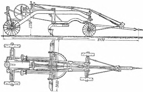
Рис. 1.11. Грейдер ГТ (1936)
