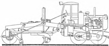
Рис. 1.21. Автогрейдер В-10 (1955)
