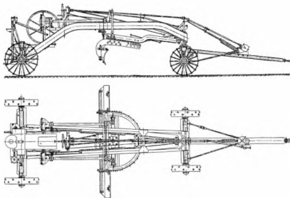
Рис. 1.14. Грейдер Д-20А (1948)
