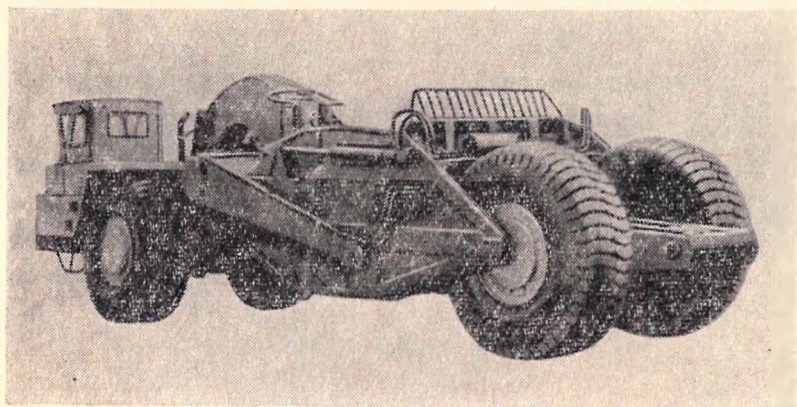
Скрепер Д-392
