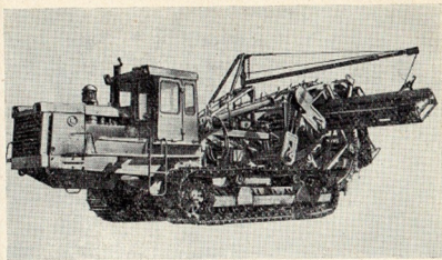
Экскаватор ЭТР-204
