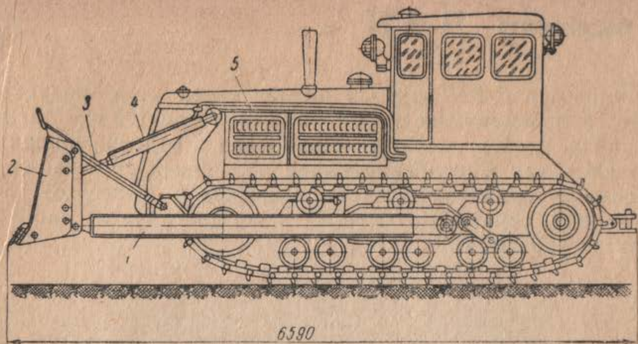
Рис. 2. Схема общего вида бульдозера Д-521:
