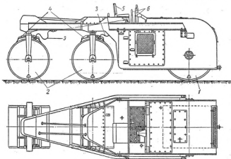
Фиг. 191б. Моторный каток трехвальный трехосный Д-178Б:
