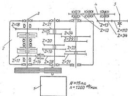
Фиг. 187. Кинематическая схема катка Д-214:
