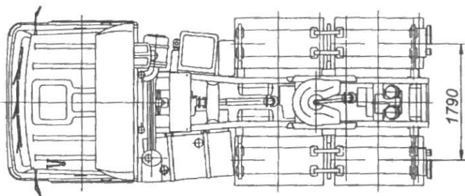
MA3 642205, 642208
