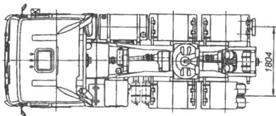
MA3 643068
