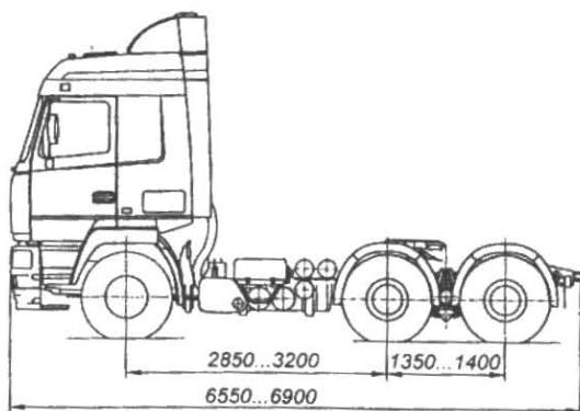
MA3 643008
