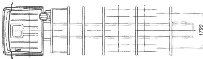
МАЗ 630300, 630305, 630306, 630307
