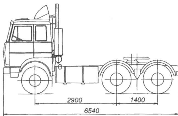
МАЗ 630300, 630305, 630306, 630307
