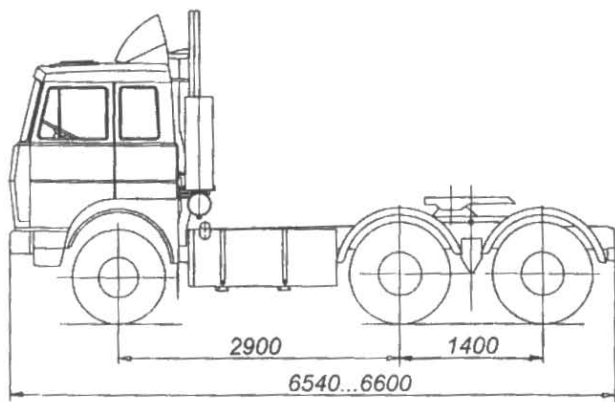
MA3 630305, 630308
