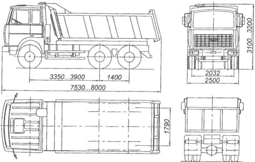
МАЗ 551600, 551603, 551606, 551656, 551605, 551650, 551607, 551657
