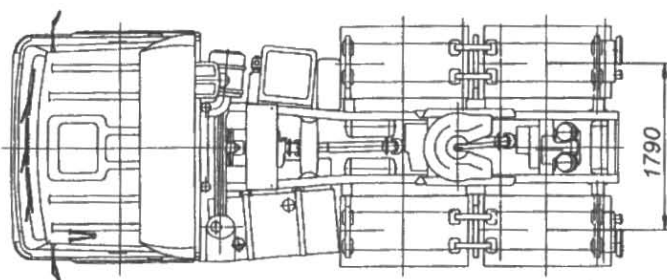
МАЗ 642205, 642290, 642296, 642297
