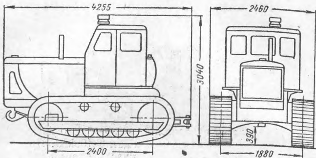
Рис. 32. Схема трактора Т-100М.
