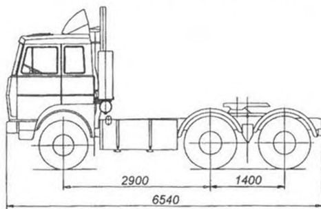
МАЗ 630300, 630305, 630306, 630307
