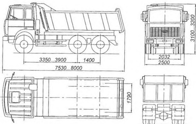
МАЗ 551600, 551603, 551606, 551656, 551605, 551650, 551607, 551657
