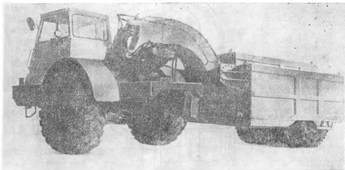
Рис. 1. Каток ДУ-16В
