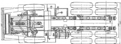
Фиг. 5. Шасси автомобиля-самосвала МАЗ-530.
