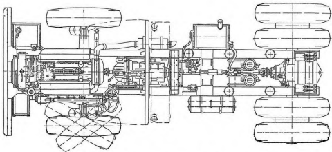
Фиг. 4. Шасси автомобиля-самосвала МАЗ-525
