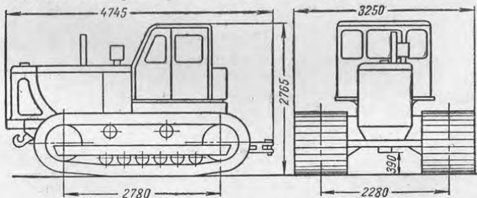
Рис. 33. Схема трактора Т-100МБ.
