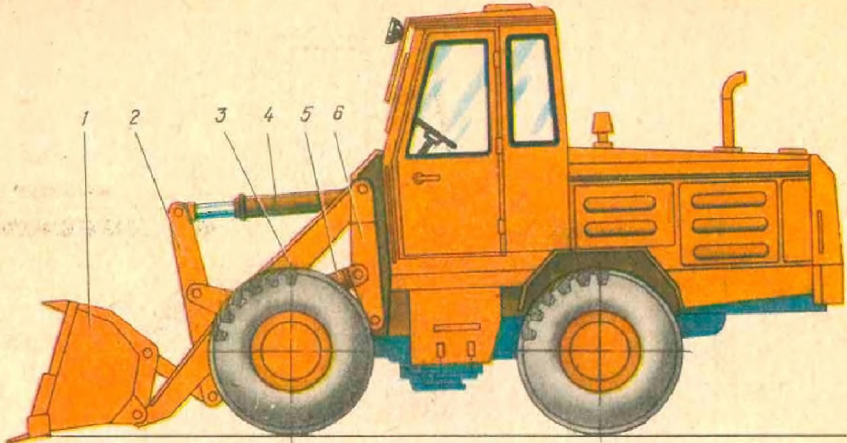
Рис. 5. Однокошковый фронтальный пневмоколесный погрузчик ТУ-6А
