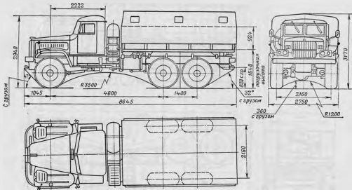
Рис. 87. Основные размеры автомобиля КраЗ-255В
