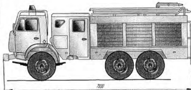
Рис.4 АЦ-4,0-40(Упан-5557)-9В
