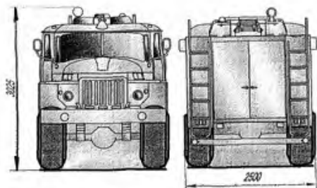
Рис.4 АЦ-4,0-40(Упан-5557)-9В
