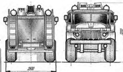
Рис.5 АЦ-5,0-40(Упан-5557)-11В
