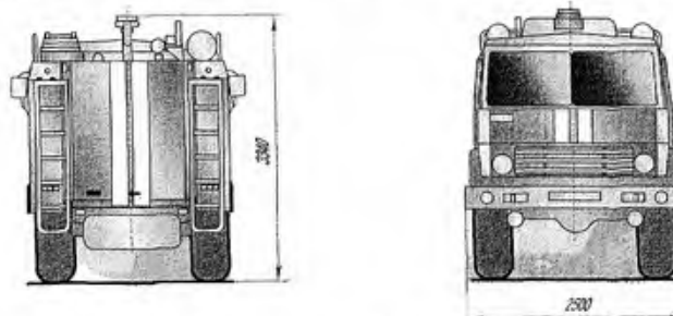
Рис.6 АЦ-5,0-40(КамАЗ-43114)-20ВР
