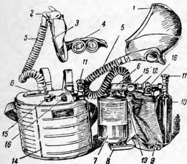
Рис. 167. Аппарат КИП-3.
