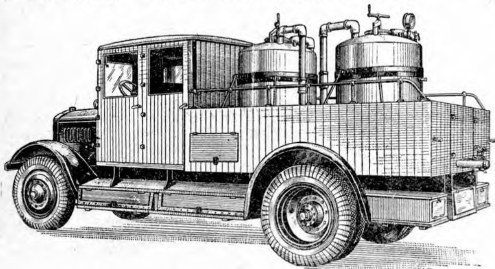
Рис. 165. Автомашина пенного огнетушения.
