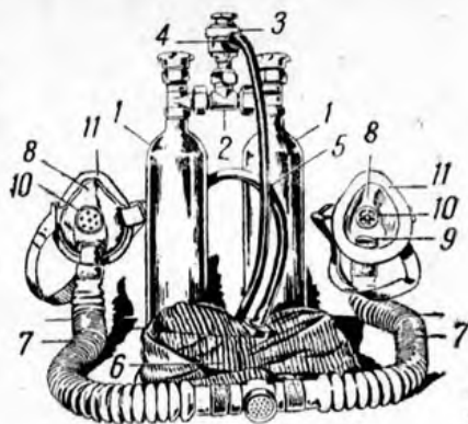
Рис. 173. Ингалятор:
