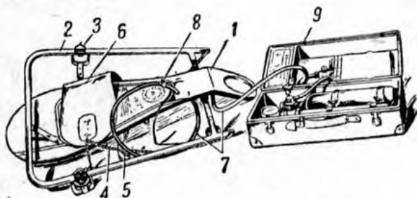
Рис. 174. Аппарат «Инхабад».
