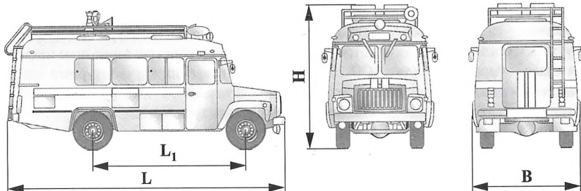
АСО-20 (ГАЗ-3308)-90ВР
