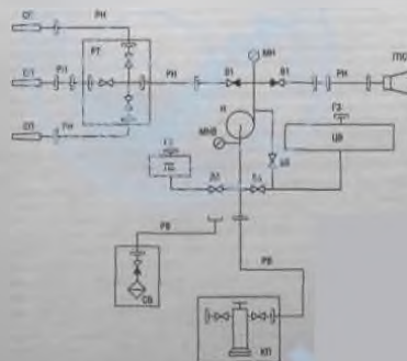
Схема водопитания насоса
