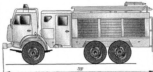
Рис. 4 АЦ-4,0-40(Упан-5557)-9Б
