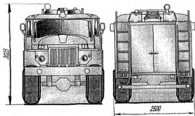
Рис. 4 АЦ-4,0-40(Упан-5557)-9Б
