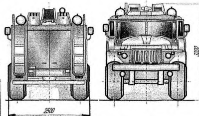
Рис. 5 АЦ-5,0-40(Упан-5557)-1Б
