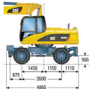
Ходовая часть с одной парой выносных опор и отвалом
