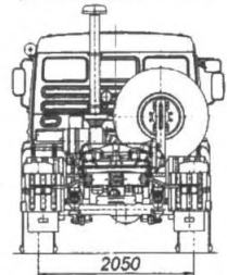
КамАЗ 44108-13
