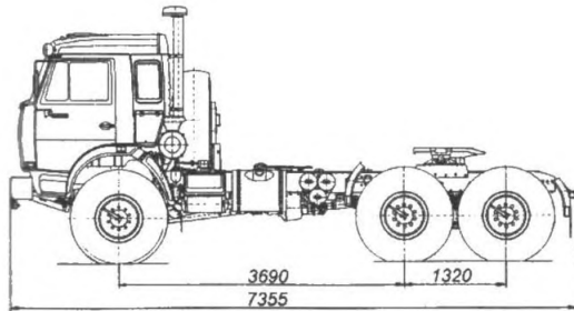
КамАЗ 43118-13
