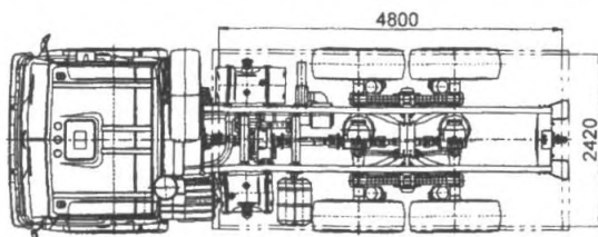
КамАЗ 43114-13, 43116-13
