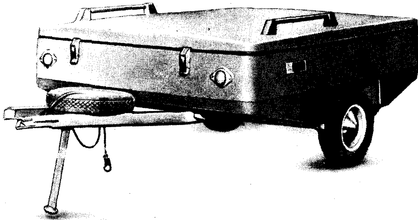
Прицеп 8106 «Скиф»
