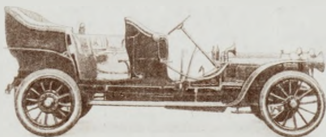
Рис. 126. "Русско-Балтийский" автомобиль с кузовом дубль-фазтон
