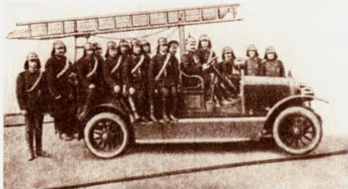
Рис. 138. Пожарный автомобиль "Русско-Балтийский" D24/40
