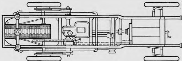
Рис. 147. Схема автомобиля с гусеницей полковника Святского
