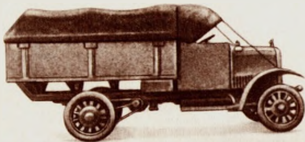
Рис. 144. 5-тонный грузовик "Русско-Балтийский" Т40/65
