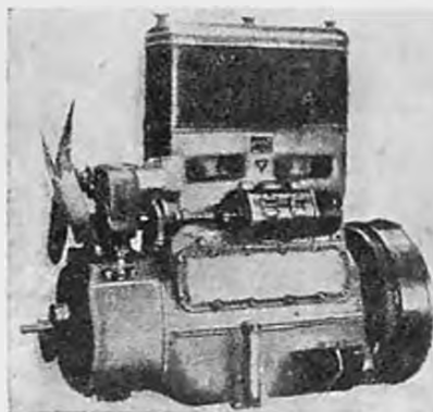
Внешний вид и разрез мотора Юнкерс-Пежо в 45 л. сил
