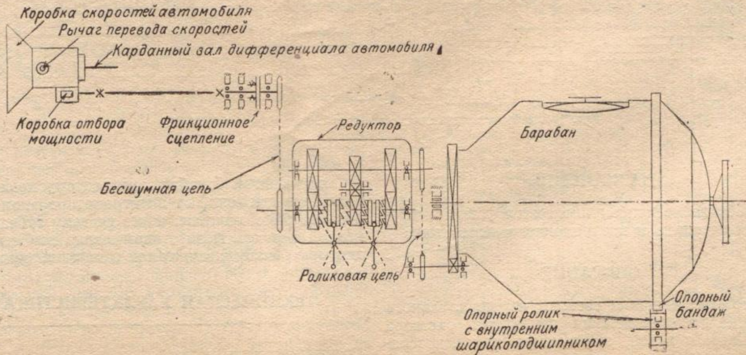
Рис. 173. Кинематическая схема привода автобетономешалки-развозки. Модель СССРМ-738 (С-49)
