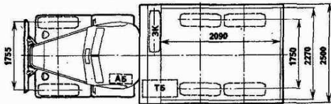
Автомобиль ЗИЛ-ММЗ-4510 6х6.1
