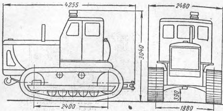
Рис. 32. Схема трактора Т-100М.
