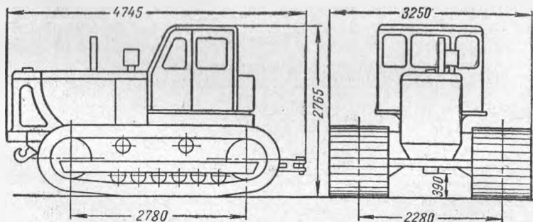
Рис. 33. Схема трактора Т-100МБ.
