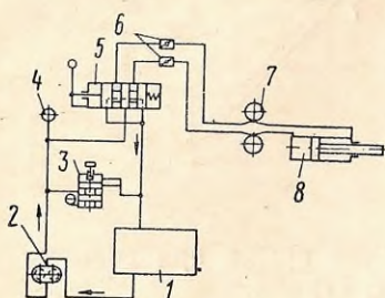
Рис. V-15. Гидравлическая система крана-трубоукладчика Т-25-50
