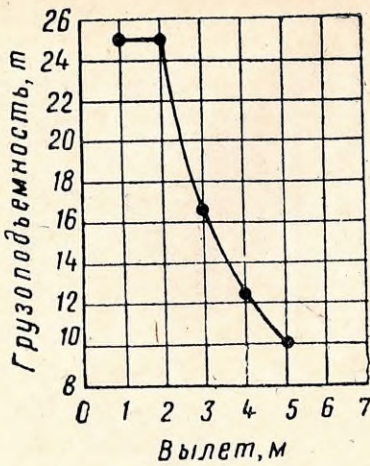
Рис. V-11. Диаграмма грузо-вых характеристик крана-тру-боукладчика Т-25-50
