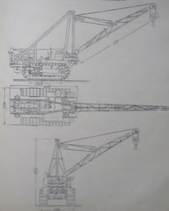
Рис. 213. Кран 2 т на тракторе «Сталинец-66».
