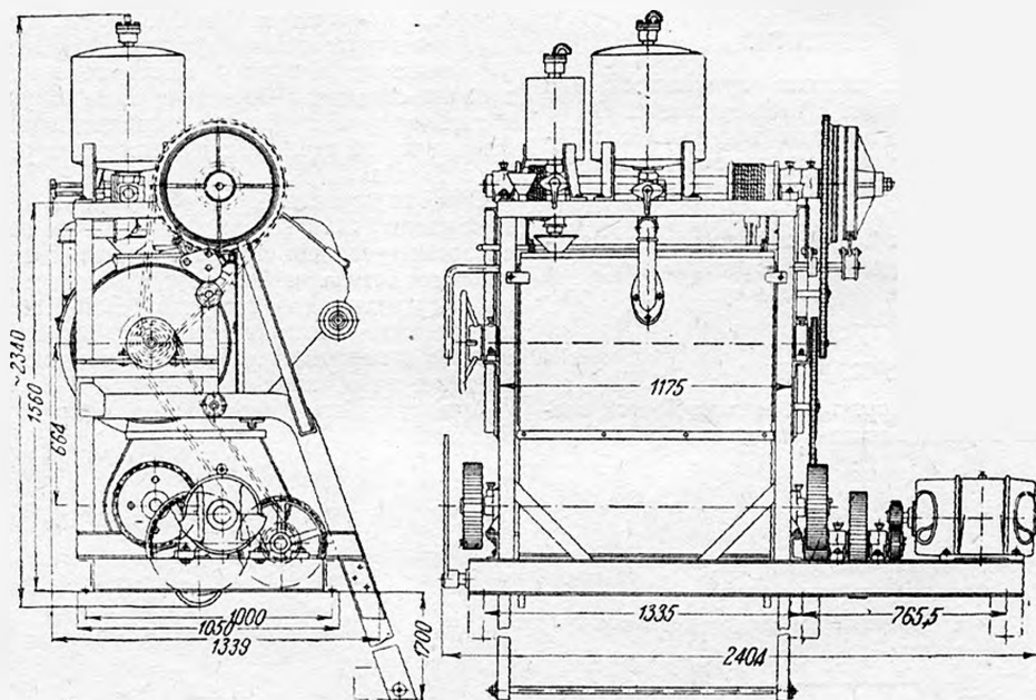
Рис. 174. Пенобетономешалка емкостью 250 л. Модель СССМ-755
