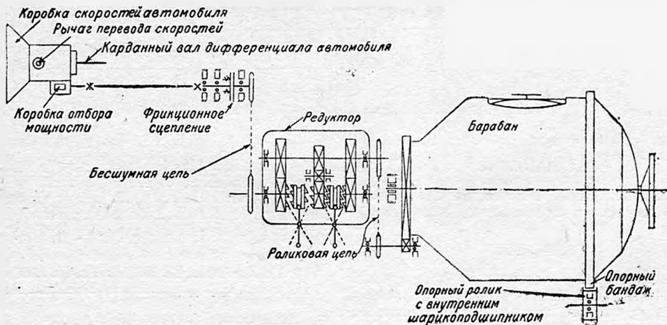
Рис. 173. Кинематическая схема привода автобетономешалки-развозки. Модель СССМ-738 (С-49)
