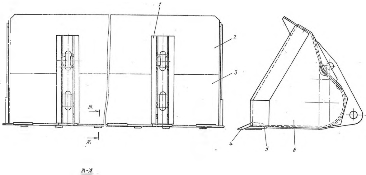
Рис. 4. Основной ковш:
