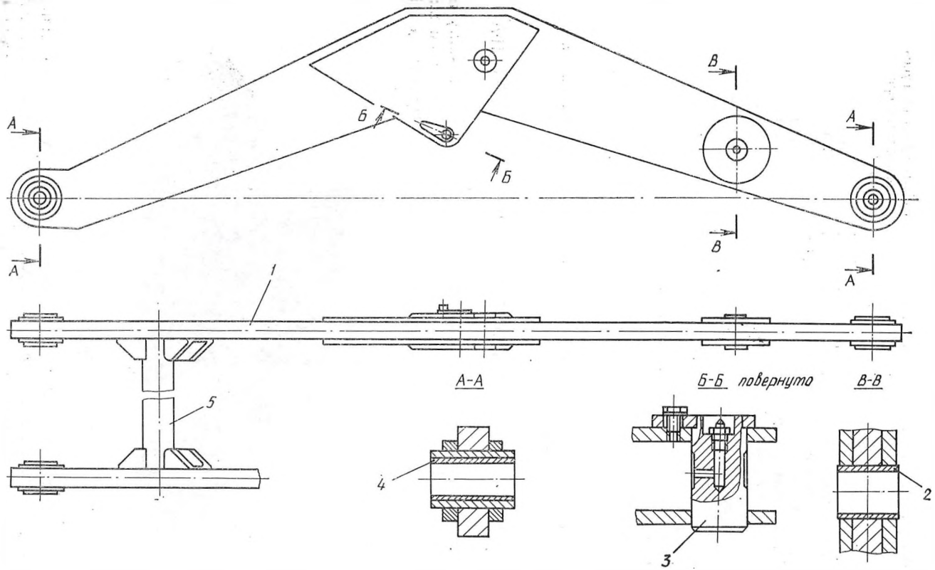
Рис. 2. Стрела: 1 — балка; 2, 4 — втулки; 3 — палец; 5 — поперечина
