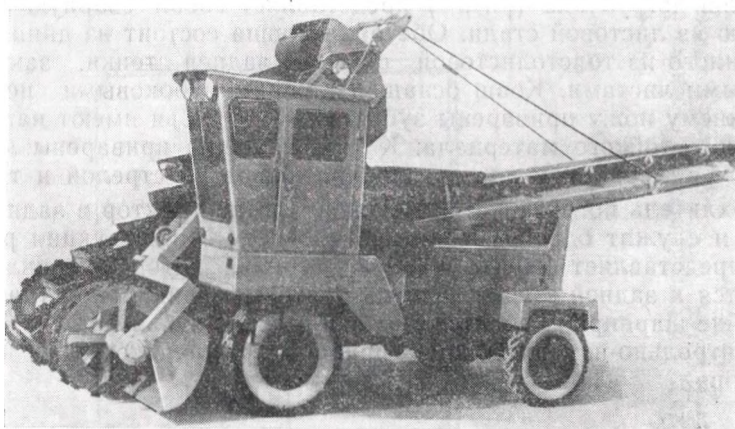
Рис. 1. Многоковшовый погрузчик ТМ-1
