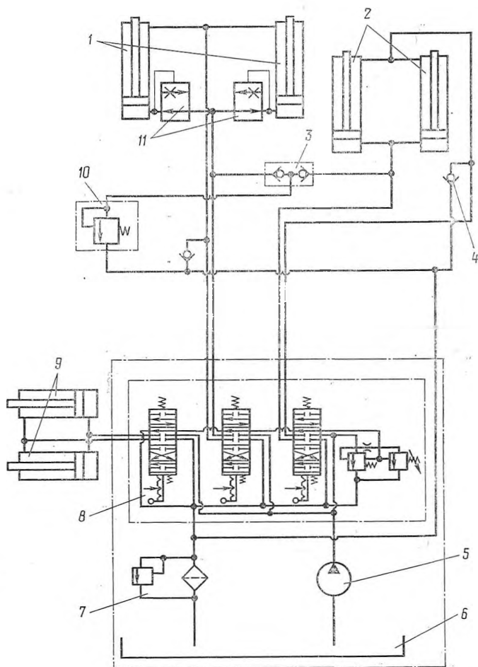
Рис. 3. Гидросистема погрузчика:
