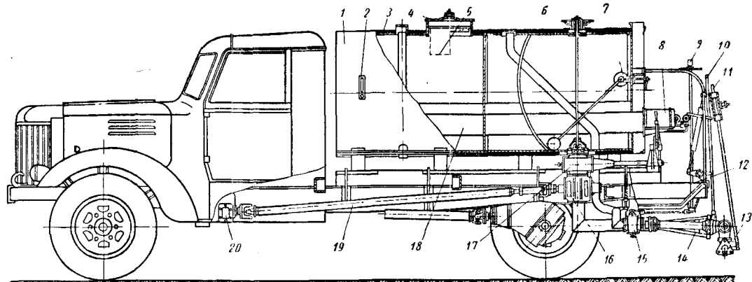
Фиг. 148. Автогудронатор Д-251: 1 — цистерна; 2 — термометр; 3 — термоизоляционный слой; 4 — люк; 5 — фильтр; 6 — запорный клапан; 7 — указатель уровня; 8 — стационарная горелка; 9 — рычаг управления разливом; 10 — рычаг сдвига распределителей; 11 — рычаг поворота распределителей; 12 — площадки; 13 — распределители; 14 — шаровое сочленение; 15 — малые краны; 16 — насос; 17 — большой кран; 18 — жаровые трубы; 19 — карданный вал; 20 — редуктор отбора мощности.
