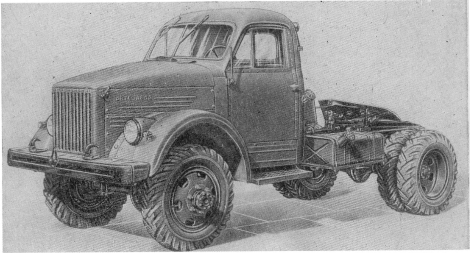
Фиг. 5. Общий вид автомобиля ГАЗ-63Д.
