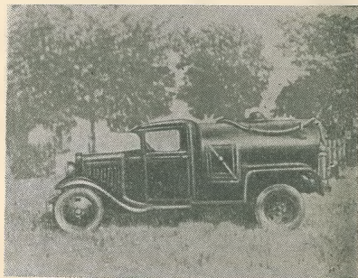
Рис. 14. Автобензозаправщик БЗ-42. Общий вид.
