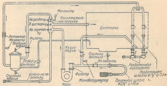
Рис. 11. Принципиальная схема БЗ-39.
