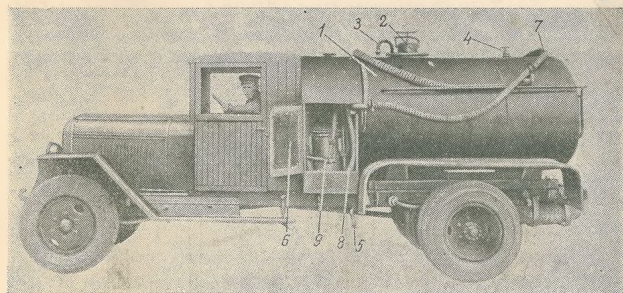
Рис. 16. Автобензозаправщик БЗ-43.
