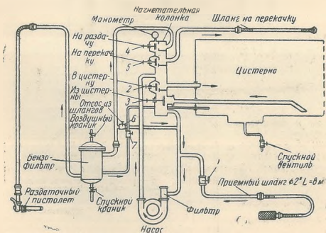
Рис. 15. Принципиальная схема БЗ-42.
