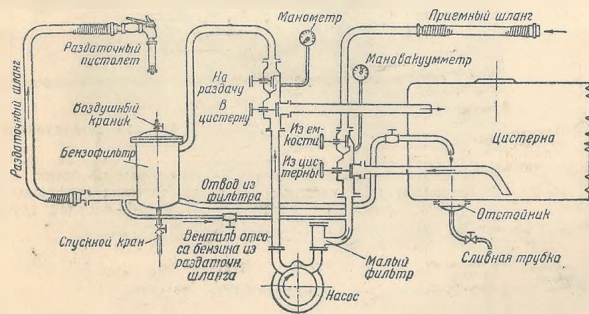
Рис. 17. Принципиальная схема БЗ-43.
