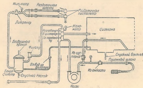
Рис. 13. Принципиальная схема БЗ-41.
