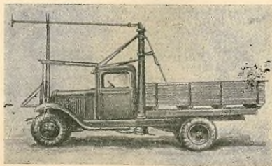
Рис. 55. Автостартер ГАЗ-АА. Общий вид:
