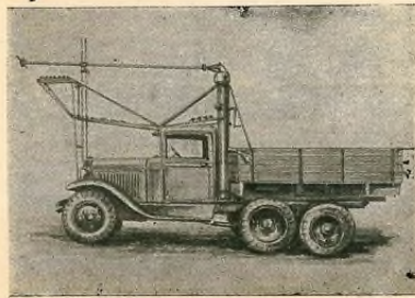
Рис. 56. Автостартер ГАЗ-ААА. Общий вид.
