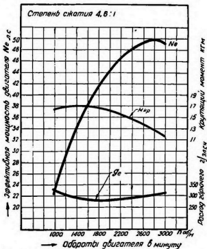
Фиг. 2. Внешняя характеристика двигателя ГАЗ-ММ.
