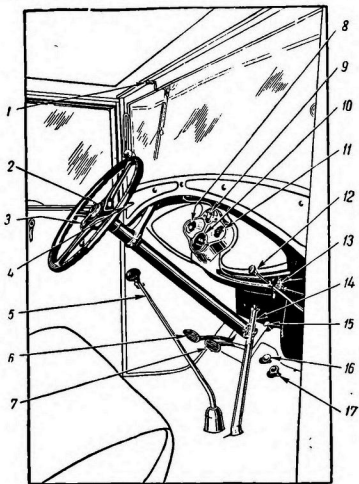
Фиг. 3. Органы управления и приборы:
