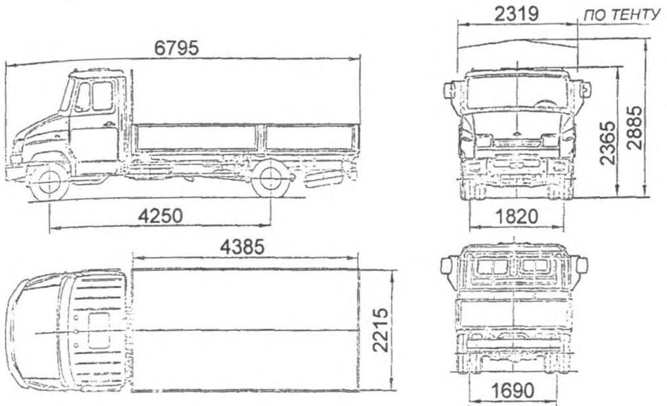
ЗИЛ 5301ДО
