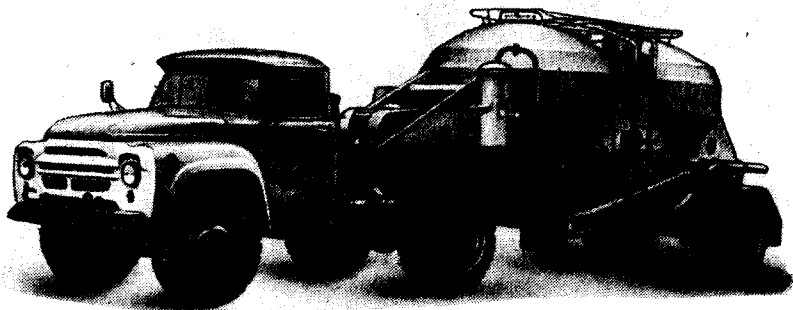
Полуприцеп-муковоз К1040-2Э с тягачом ЗИЛ-130В1
