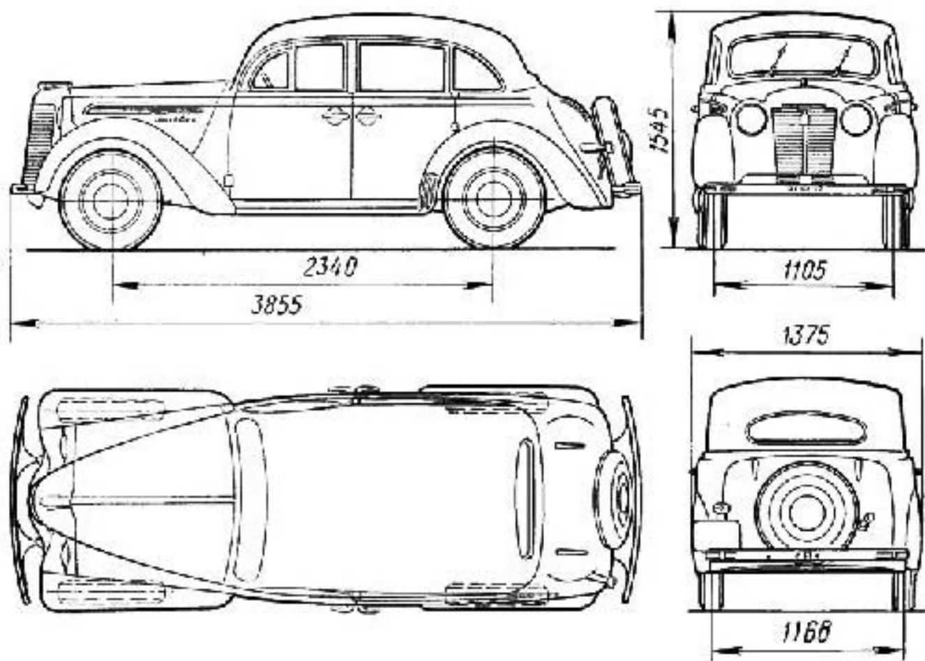
Технические характеристики Москвича М-400-420
